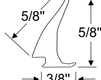
WHITE RUBBER 70-4771-257 per/ft.
