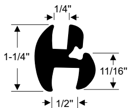
70-4774-257 • per/ft. USES 60-0607-257 LOCKSTRIP
