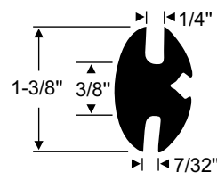
70-4299-257 • per/ft. USES 60-0607-257 LOCKSTRIP
